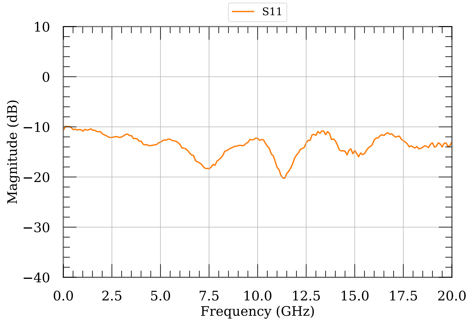
LNA S-params module052
